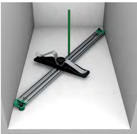
Find body and door centre lines Korpus- und Türmitte finden
